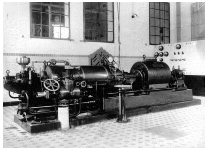
Erste BBC-Dampfturbine, 1901
